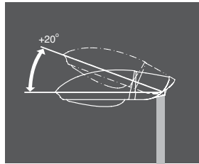
قابلیت تنظیم زاویه نصب چراغ تا ۱۰- درجه در حالت نصب افقی و ۲۰- درجه در حالت نصب عمودی
