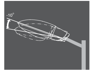
قابلیت تنظیم زاویه نصب چراغ تا ۱۰- درجه در حالت نصب افقی و ۲۰- درجه در حالت نصب عمودی
