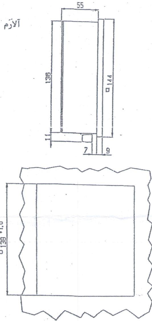
ابعاد برش بر روی تابلو جهت نصب رگولاتور
