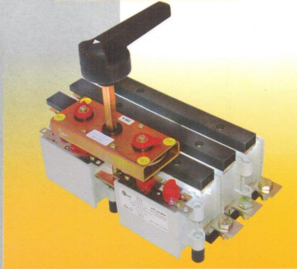
کلید دو طرفه دسته معمولی
