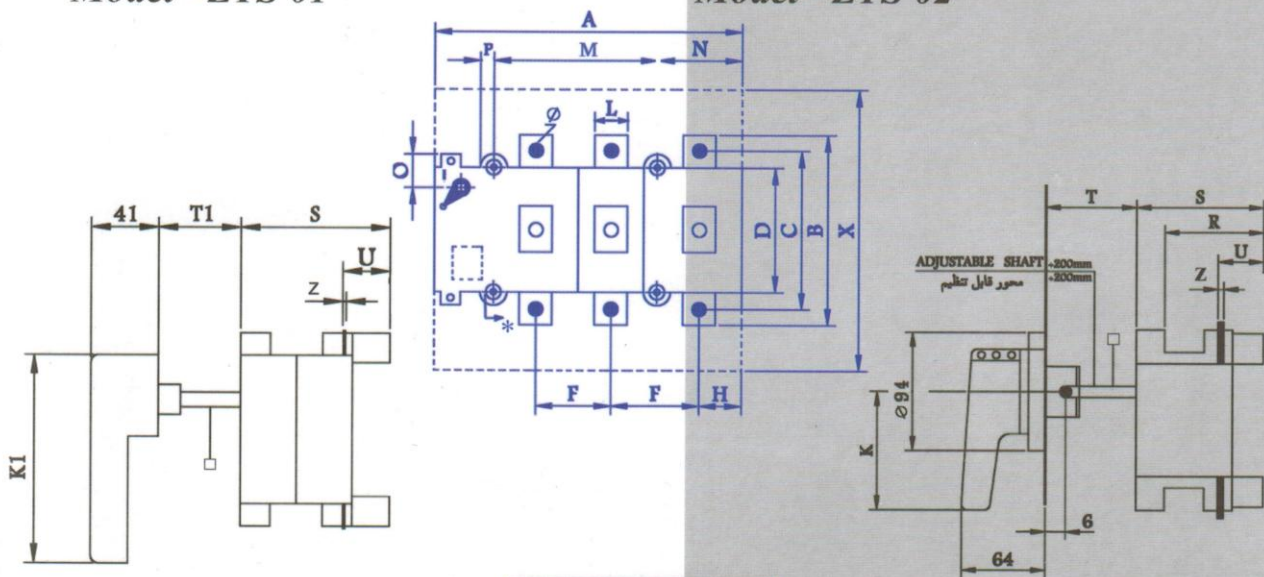
ابعاد کلی کلید های مدل ZTS Overall dimensions switches/ZTS
